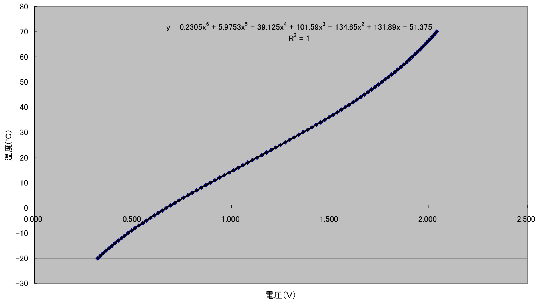
電圧(中間電圧V0)と温度(°C)の近似式
